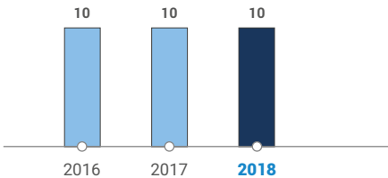
Прямые выбросы парниковых газов 1 (Scope 1, млн т)
